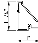
1"X1 1/4" SNAP TRIM M20546 - BASE CLIP M20545 - TRIM
